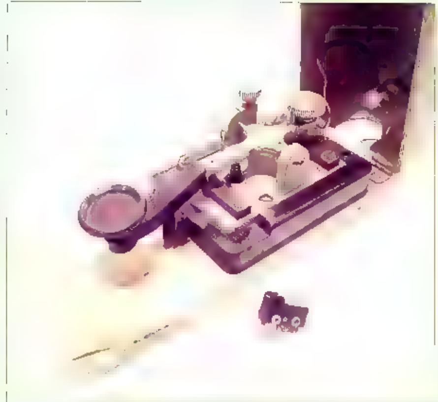
Deze junker is al zeker 60 jaar oud en gebruikt bij de Duitse Marine tijdens de Tweede Wereldoorlog. Wie de huidige junker kent ziet dat er in al die jaren weinig is veranderd... behalve de kleur.
